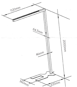
ABMESSUNGEN
