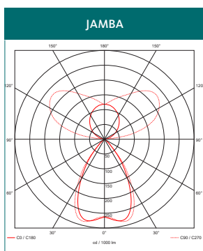
LICHTVERTEILUNG
